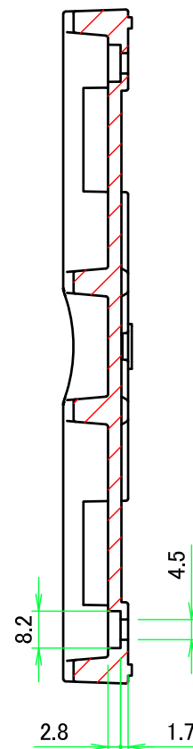
A-A ( 1 : 1.5 )
